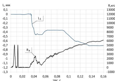
Рис. 4. Криві залежності тяги R_x та переміщення рухомої частини стапеля L_1 від часу в момент виходу двигуна № 2 на основний режим під час випробування № 3
