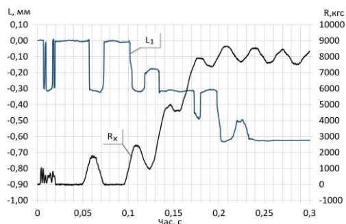
Рис. 4. Криві залежності тяги R_x та переміщення рухомої частини стапеля L_1 від часу в момент виходу двигуна № 2 на основний режим під час випробування № 3
