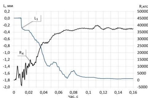
Рис. 5. Криві залежності тяги R_x та переміщення рухомої частини стапеля L_1 від часу в момент виходу двигуна № 3 на основний режим: а – під час випробування № 1; б – під час випробування № 2
