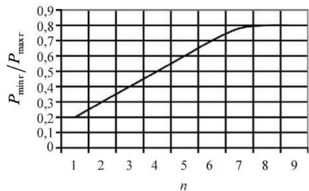
Рис. 3. Графік n = f\left(\frac{P_{\text{minг}}}{P_{\text{maxг}}}\right)
