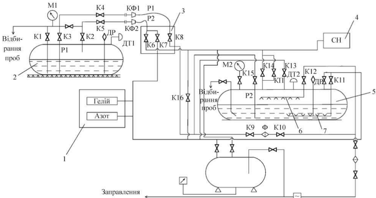
Рис. 1. Спрощена пневмогідролічна схема зливання палива:
