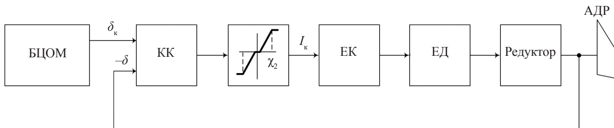
Рис. 1. Структурна схема слідкувального електропривода:
