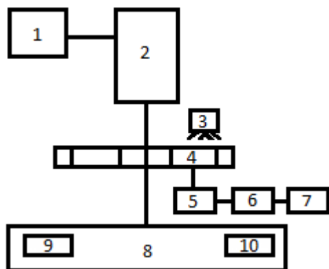
Рис. 1. Структурная схема: 1 – пульт управления; 2 – электрический двигатель; 3 – источник света; 4 – диск-модулятор с 60 отверстиями; 5 – фотоприемник; 6 – плата форми- рования импульсов; 7 – частотомер; 8 – ротор; 9 – испытуемый узел; 10 – противовес
