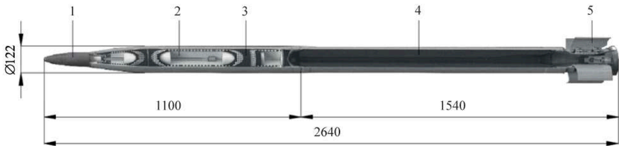
Рис. 5. 122-міліметровий некерований реактивний снаряд 9М538:
