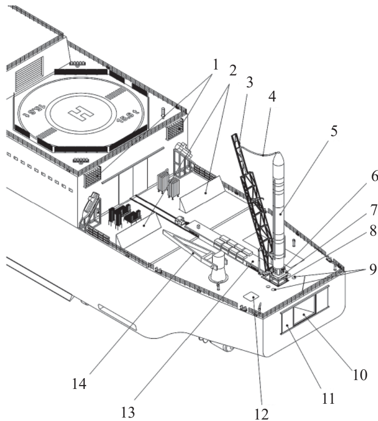
Рис. 5. Пускове судно. Кормова частина. Технологічне обладнання та РКП на момент пуску:
