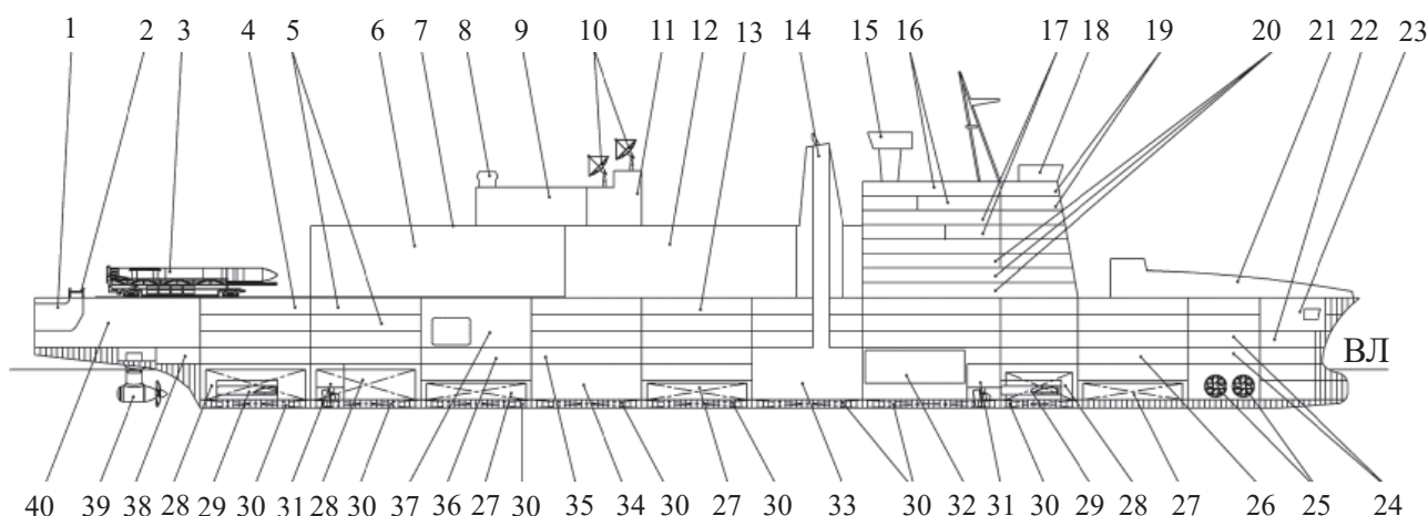
Рис. 3. Пускове судно. Поздовжній переріз:
