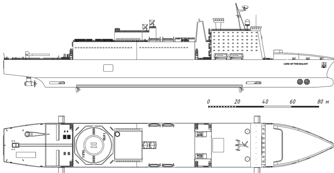
Рис. 2. Пускове судно. Вигляд з правого борту та зверху
