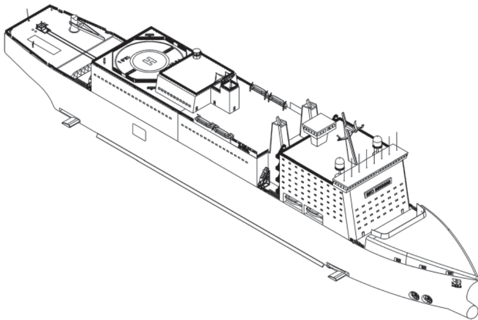
Рис. 1. Пускове судно. Загальний вигляд
