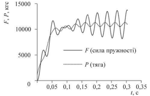
Рис. 6. Перший випадок – частота пульсації тяги дорівнює частоті поступальних коливань (резонанс)
