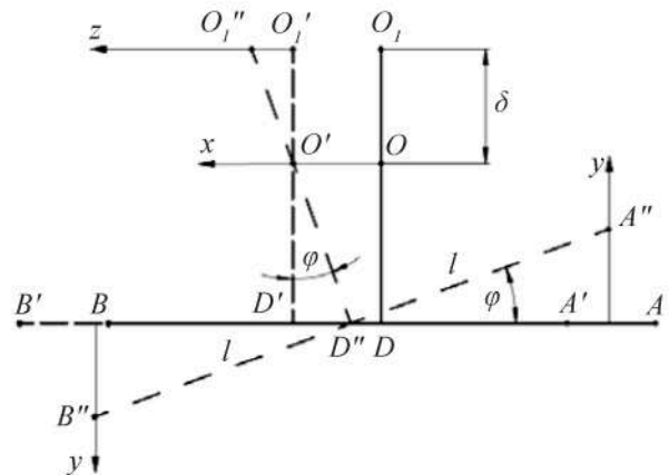
Рис. 4. Схема зміщення системи
