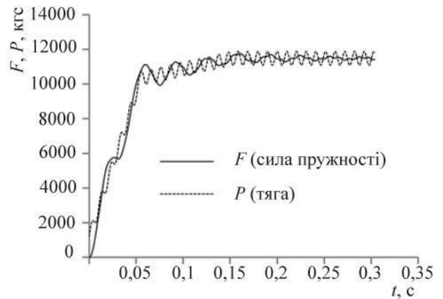
Рис. 7. Другий випадок – частота пульсації тяги дорівнює частоті обертальних коливань
