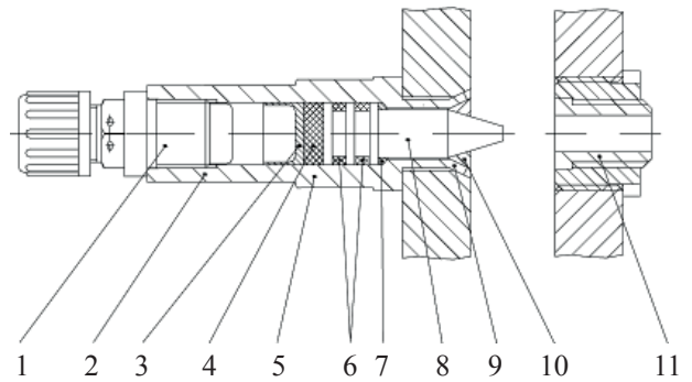
Рис. 4. Піроболт після спрацьовування
