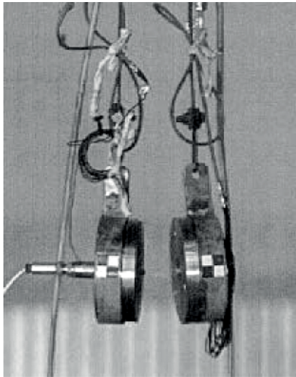
Рис. 7. Маятниковий підвіс з роз'єднаними фланцями після спрацьовування піроболта
