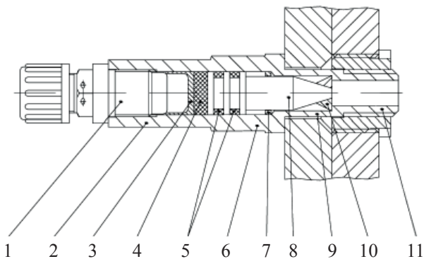
Рис. 3. Піроболт до спрацьовування
