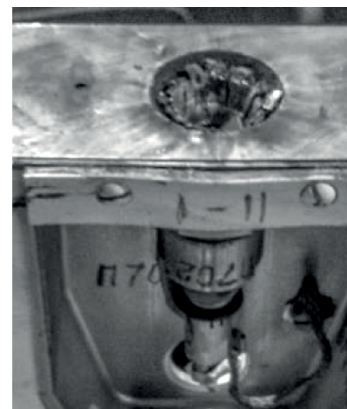
Рис. 2. Місце встановлення розривного болта РБ16М у шпангоуті міжступеневого відсіку РН «Циклон-4»
