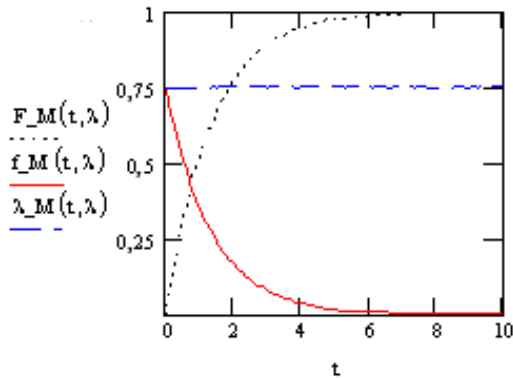
Рис. 1. Приклад графіка: F_M(t, \lambda) і f_M(t, \lambda) – функція і щільність розподілу інтервалу часу між подіями у потоці; \lambda_M(t, \lambda) – інтенсивність подій у потоці; \lambda = 0,75
